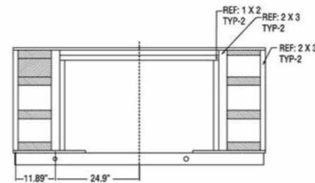
Pohľad na prednú stranu rámu
