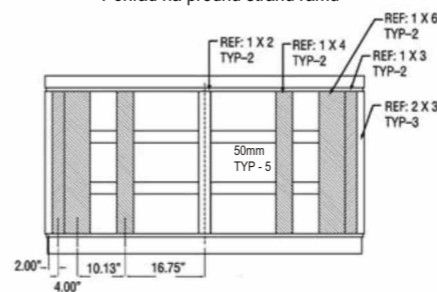
Pohľad na bočnú stranu rámu
