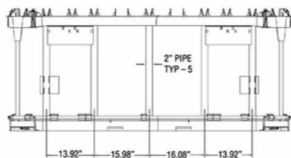
Pohľad na zadnú stranu rámu
